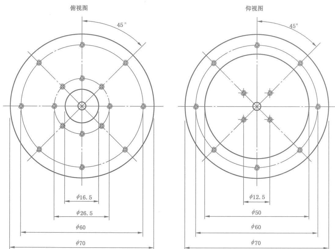
图 C.1 同轴靶的机械图
