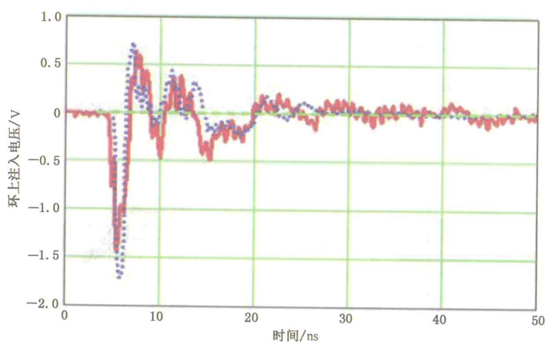
图 D.6 在距离环 45 cm 处的电压降实测(实线)和数值仿真(点线)的比较(感应电压)
