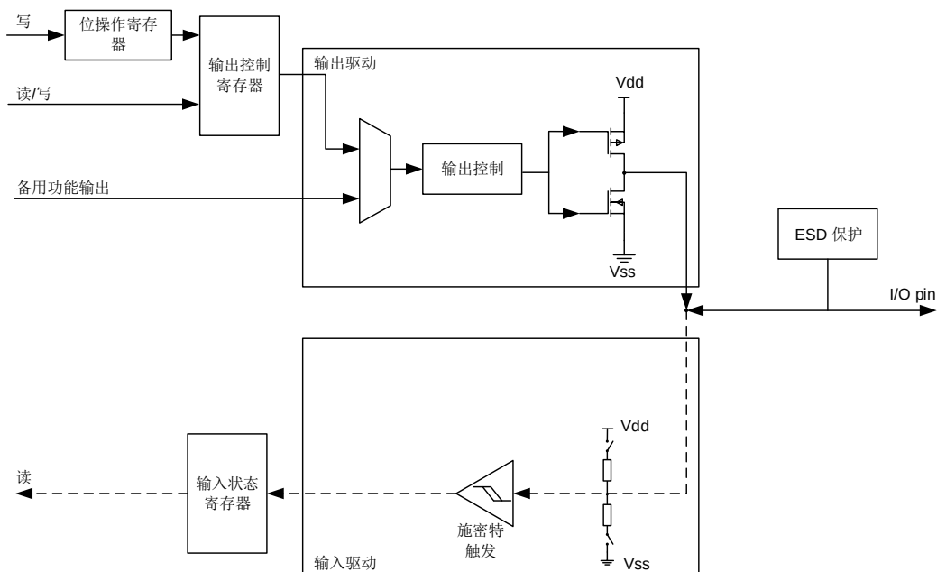
图 7-3. 输出配置
