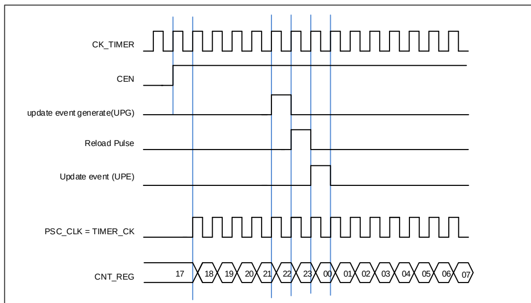
图 15-54. 内部时钟分频为 1 时正常模式下的控制电路
