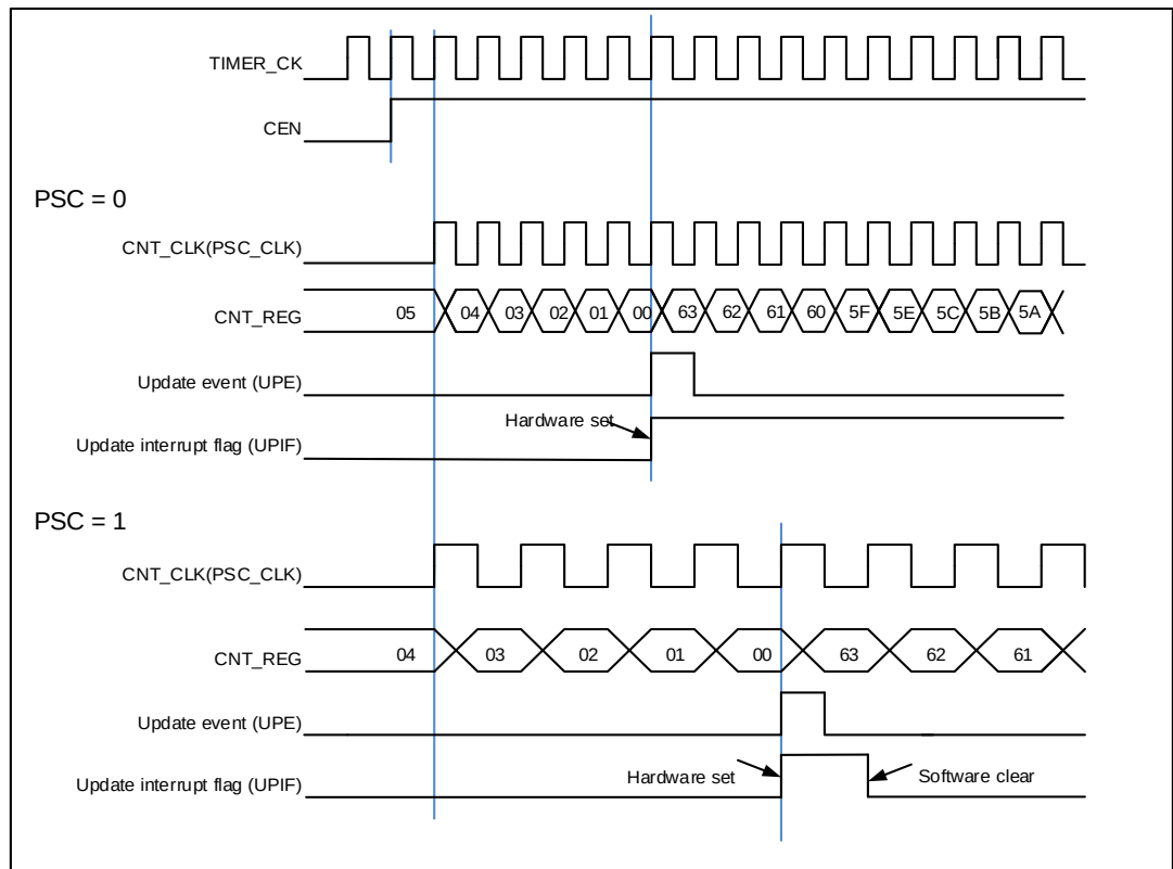
图 15-58. 向下计数时序图, PSC=0/1
