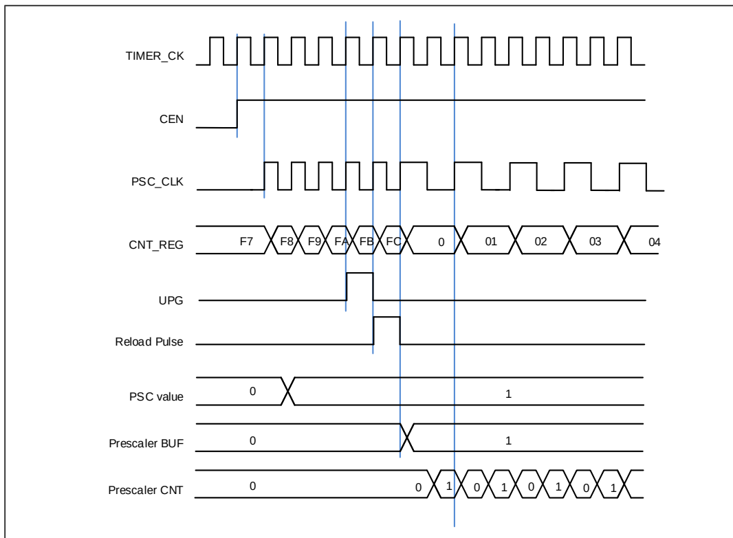
图 15-82. 当预分频器的参数从 1 变到 2 时，计数器的时序图
