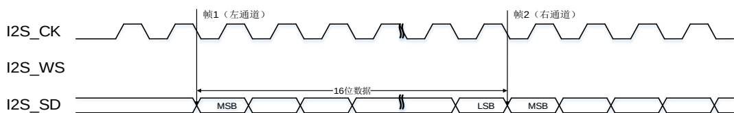
图 18-8. I2S 飞利浦标准时序图（DTLEN=00, CHLEN=0, CKPL=0）
