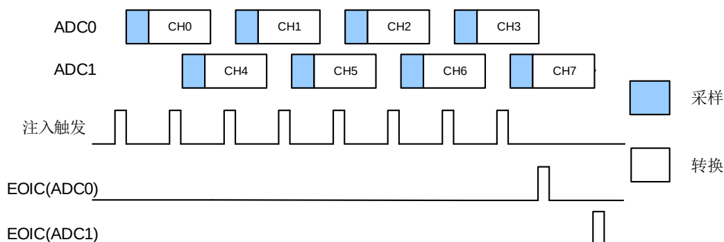
图 11-16. 交替触发: 间断模式下注入通道组
