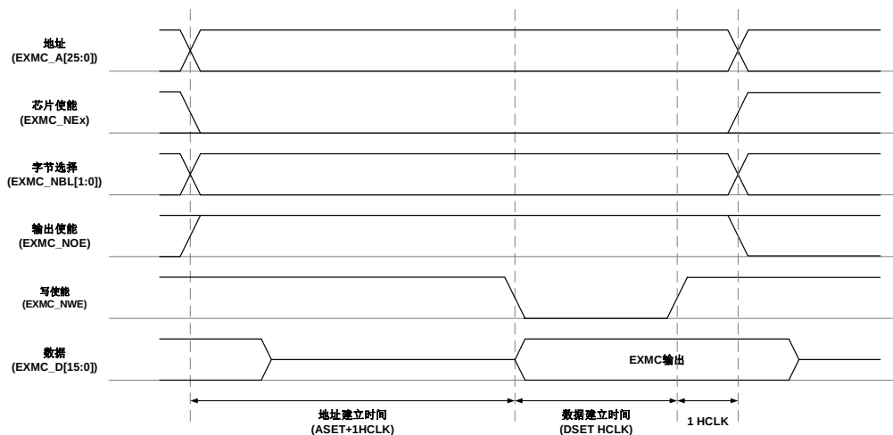
图 20-7. 模式 1 写时序
