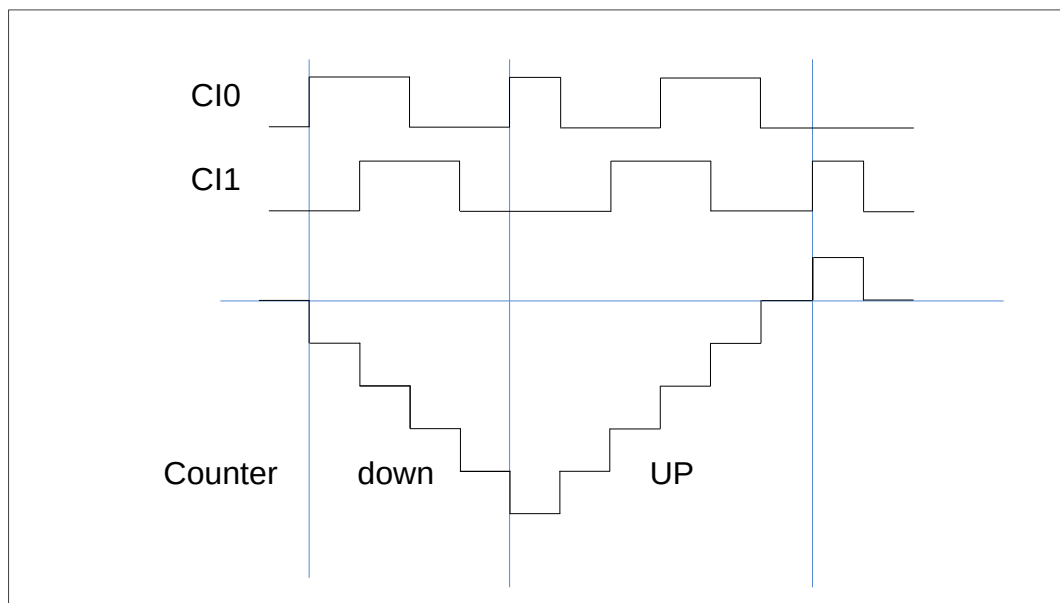
图 15-48. CI0FE0 极性反相的编码器接口模式下的例子
