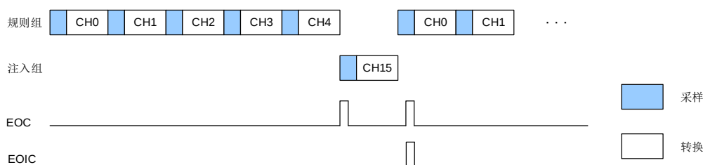
图 11-7. 自动注入，CTN=1
