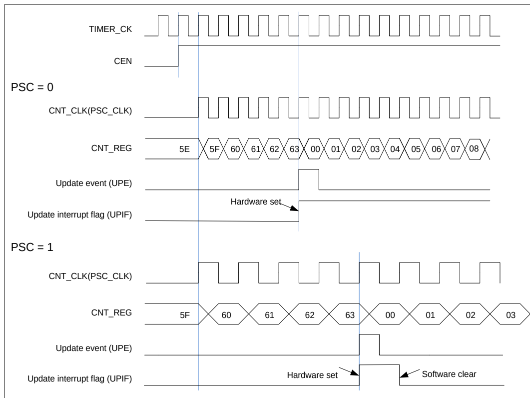
图 15-4. 向上计数时序图, PSC=0/1
