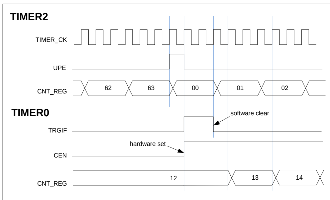
图 15-30. 用定时器 2 的更新事件来启动定时器 0
