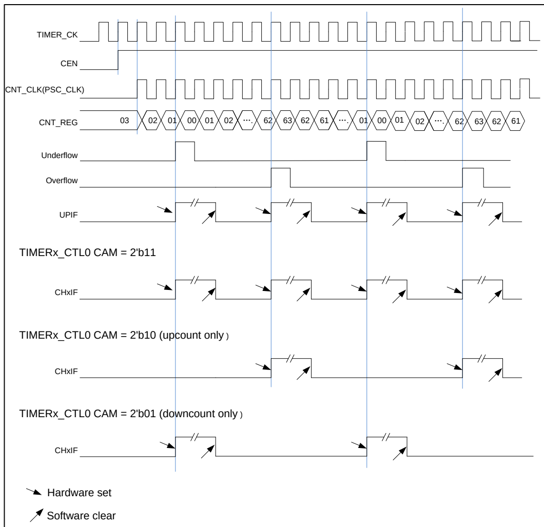
图 15-77. 中央对齐计数模式计数器时序图
