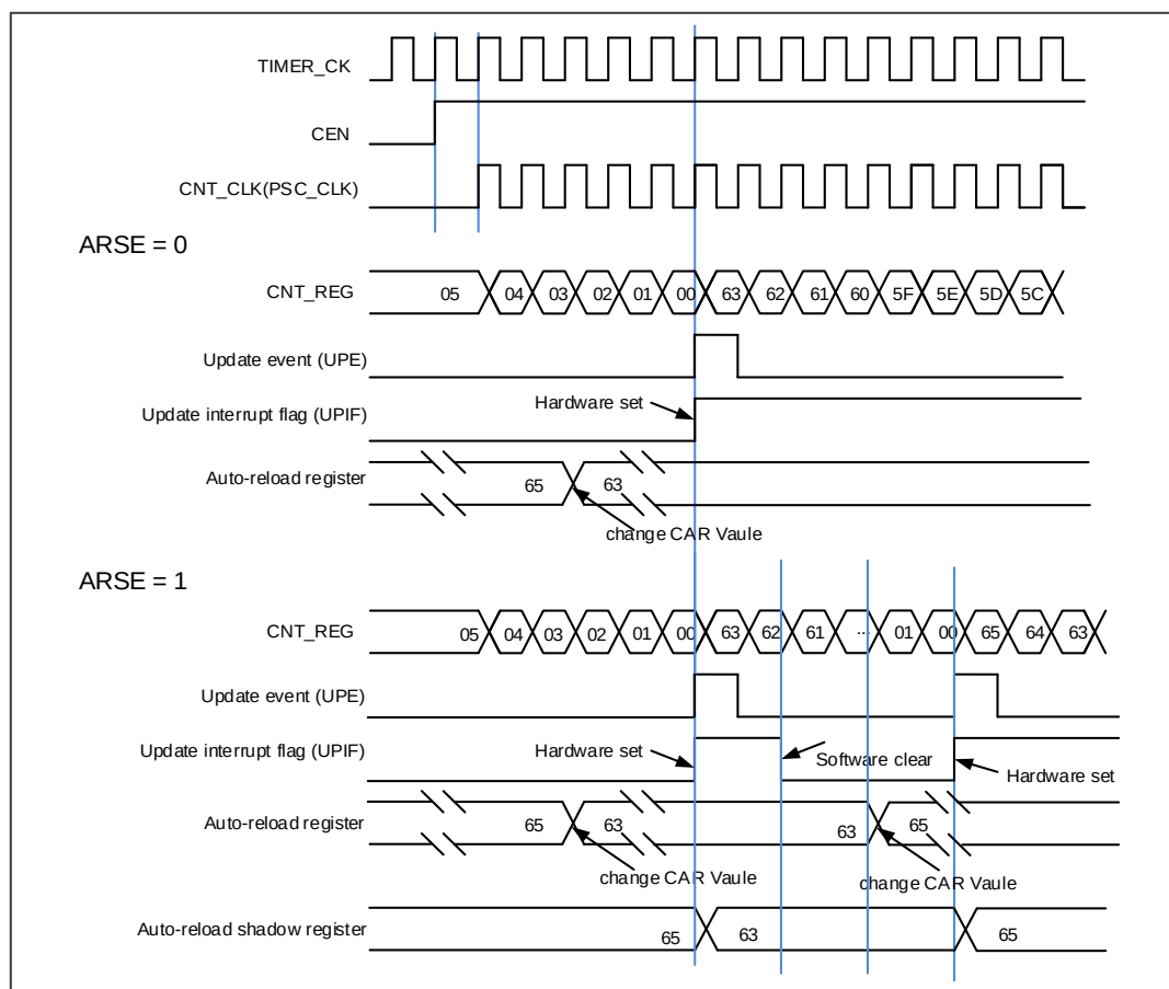
图 15-40. 向下计数时序图，在运行时改变 TIMERx_CAR 寄存器值
