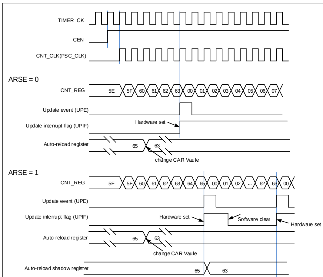
图 15-74. 向上计数时序图，在运行时改变 TIMERx_CAR 寄存器的值
