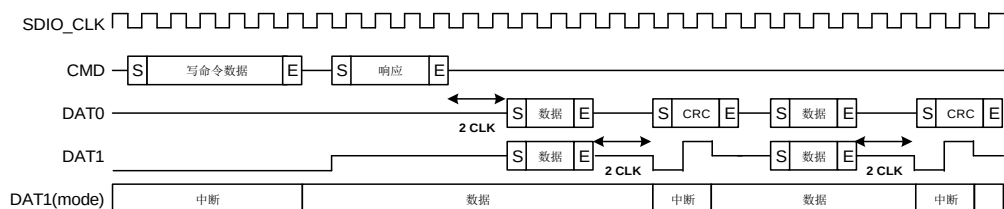
图 19-18. 4 位模式下多块写中断周期时序
