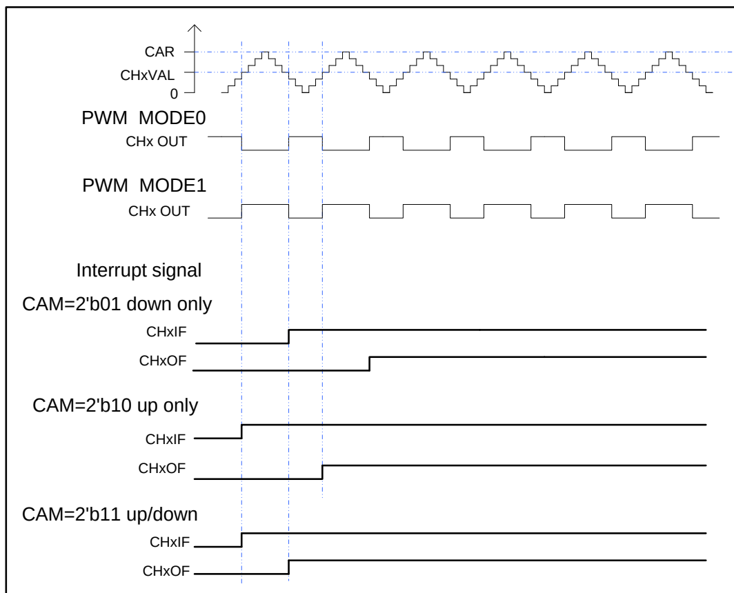
图 15-17. CAPWM 时序图
