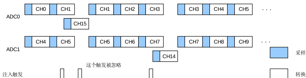
图 11-18. 在注入转换过程中触发出现
