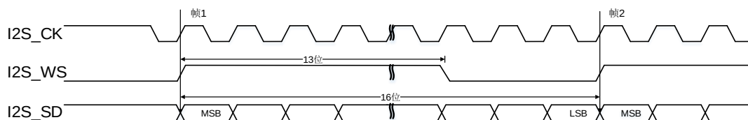
图 18-37. PCM 标准长帧同步模式时序图 (DTLEN=00, CHLEN=0, CKPL=1)
