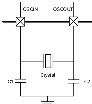
图5-7. HXTAL时钟源
