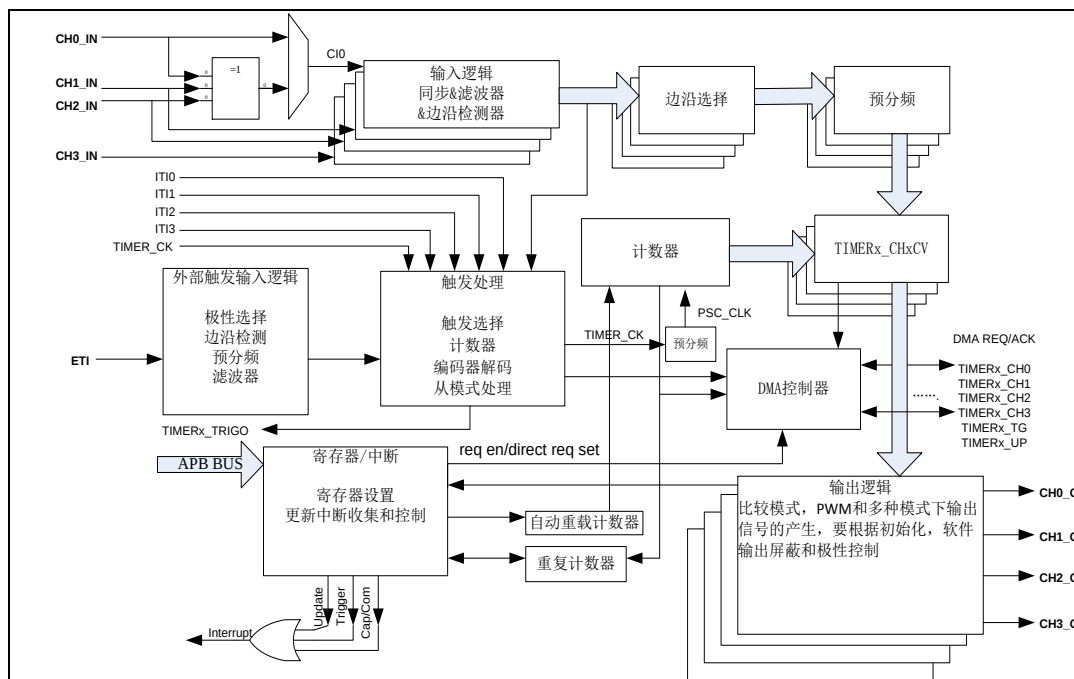
图 15-34. 通用定时器 L0 结构框图
