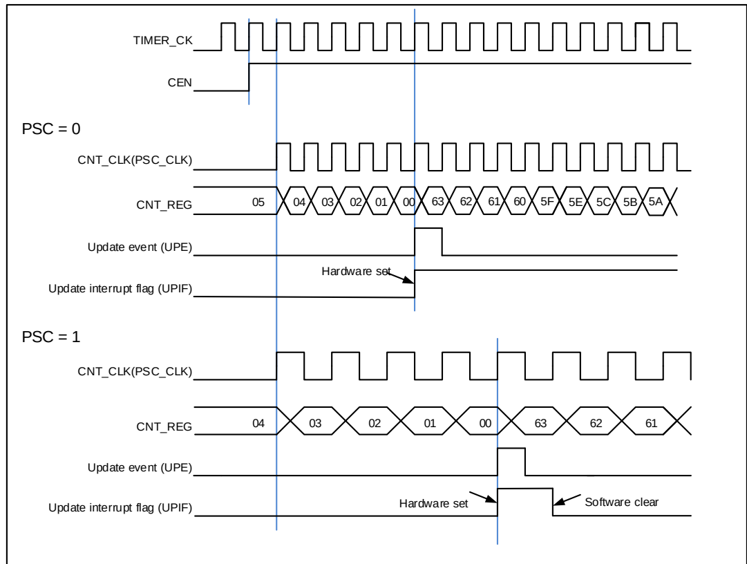
图 15-39. 向下计数时序图, PSC=0/1
