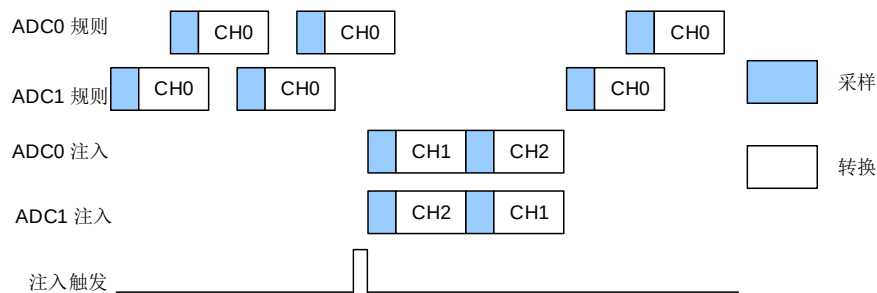
图 11-19. 交叉的单通道转换被注入序列 CH1 和 CH2 中断
