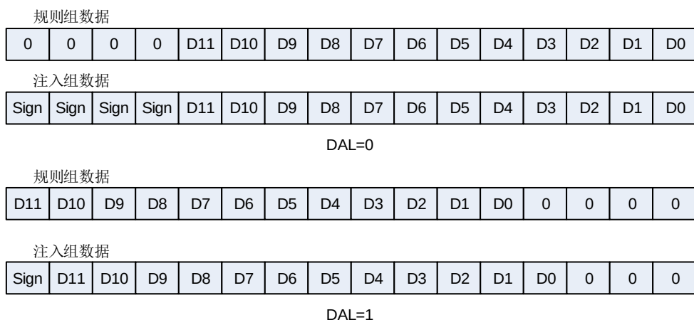
图 11-9. 12 位数据对齐
