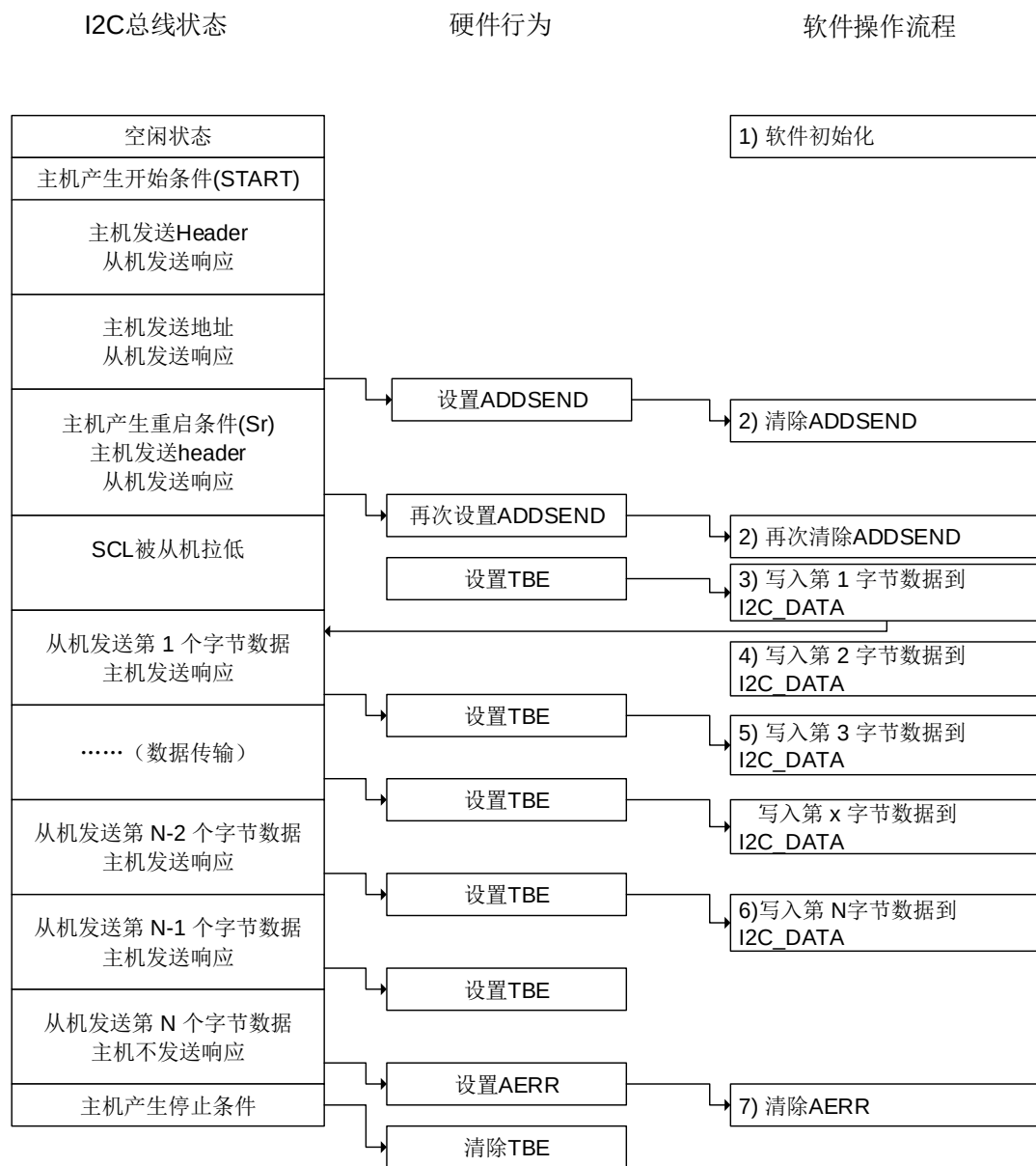
图 17-9. 从机发送模式（10 位地址模式）
