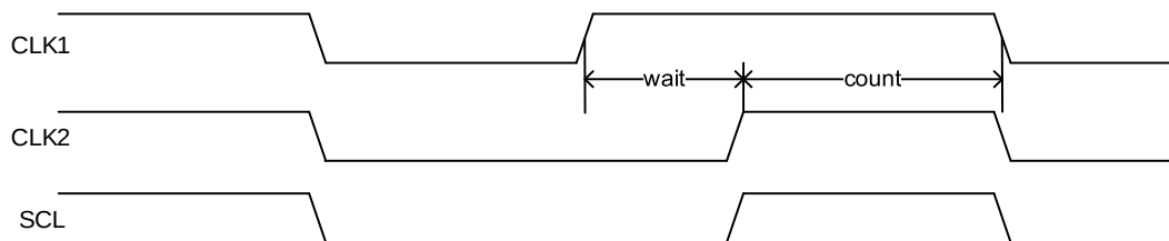
图 17-4. 时钟同步
