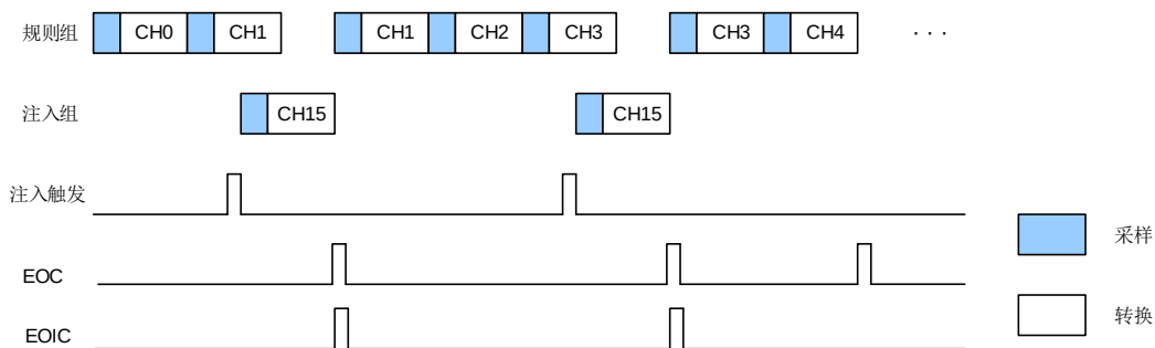
图 11-8. 触发注入
