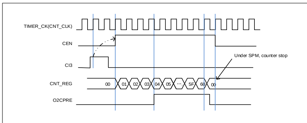
图 15-27. 单脉冲模式，TIMERx_CHxCV = 0x04，TIMERx_CAR=0x60
