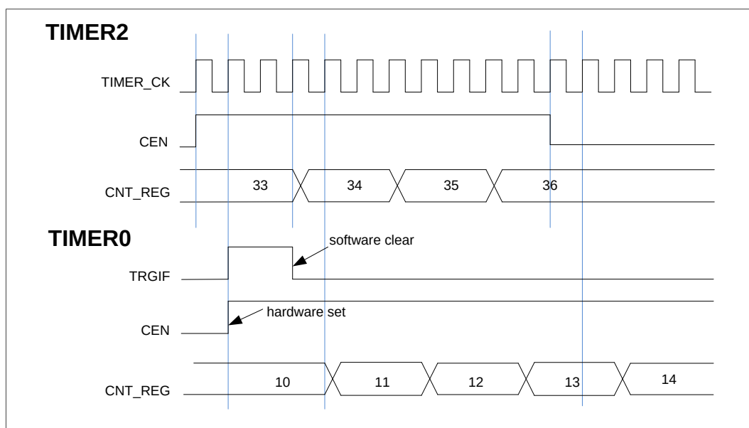
图 15-29. 用定时器 2 的使能信号启动定时器 0
