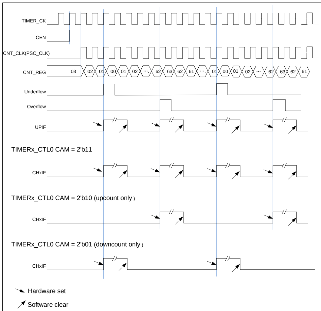
图 15-60. 中央对齐计数模式计数器时序图
