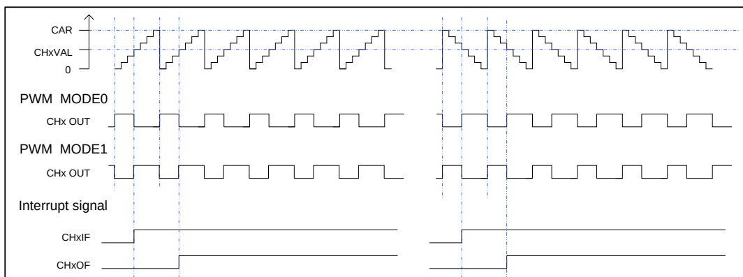
图 15-65. CAPWM 时序图
