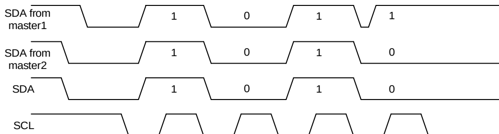
图 17-5. SDA 线仲裁
