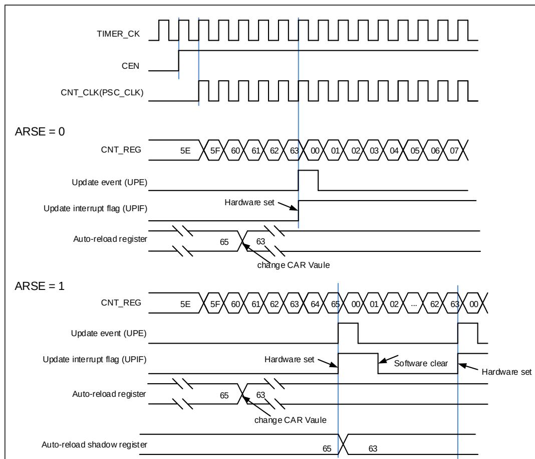
图 15-57. 向上计数时序图，在运行时改变 TIMERx_CAR 寄存器的值
