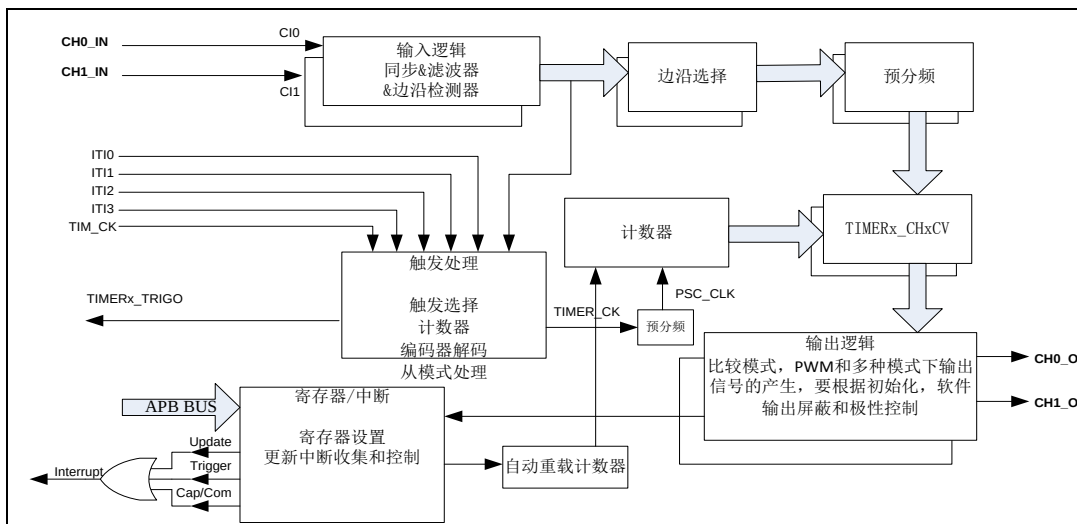
图 15-53. 通用定时器 L1 结构框图
