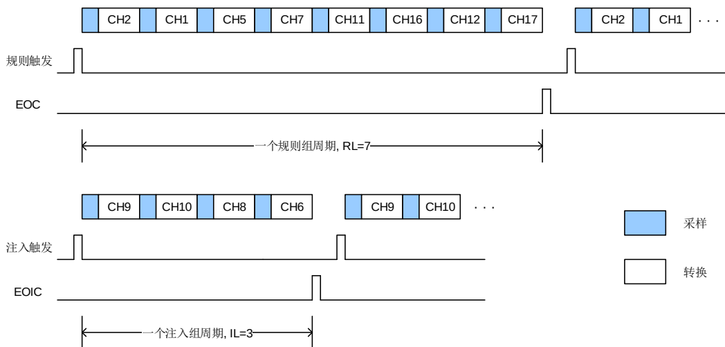
图 11-4. 扫描转换模式，且连续转换模式禁能
