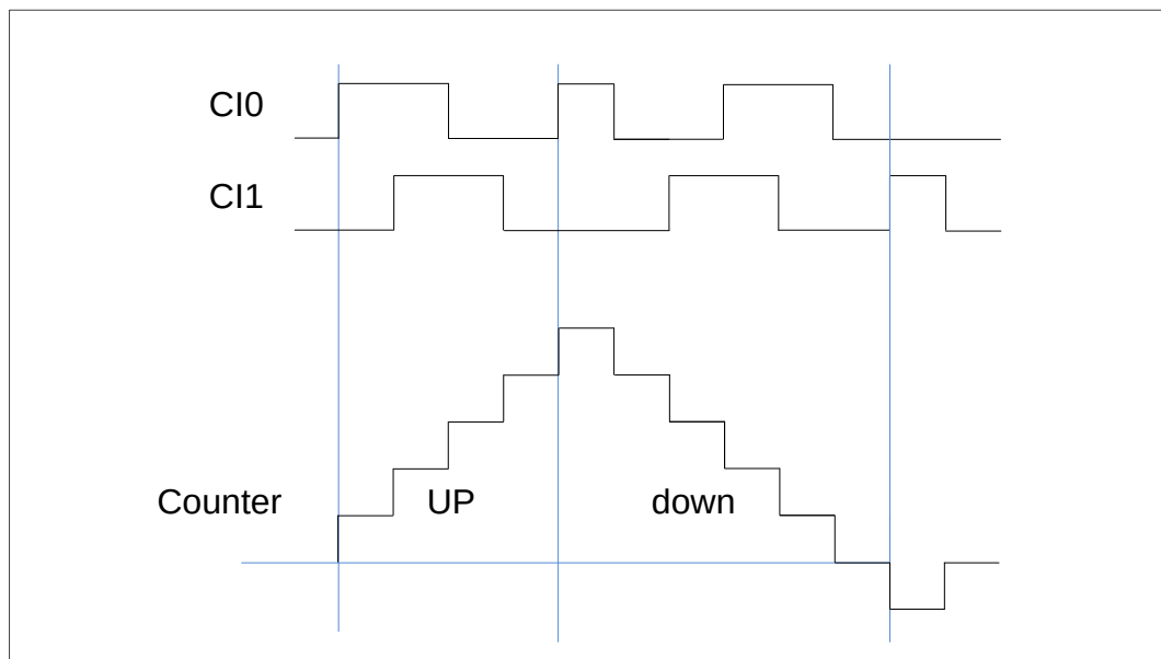
图 15-47. 编码器接口模式下计数器运行例子
