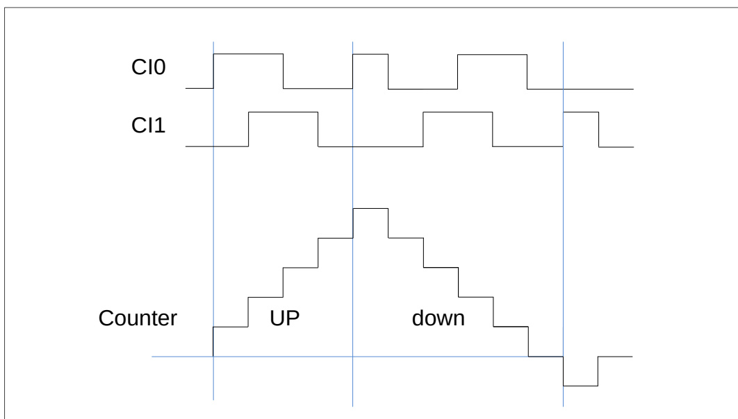
图 15-20. 编码器接口模式下计数器运行例子
