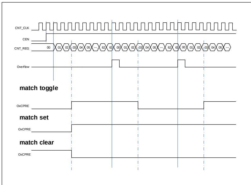
图 15-63. 三种输出比较模式
