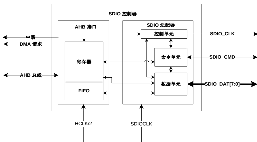
图 19-6. SDIO 框图
