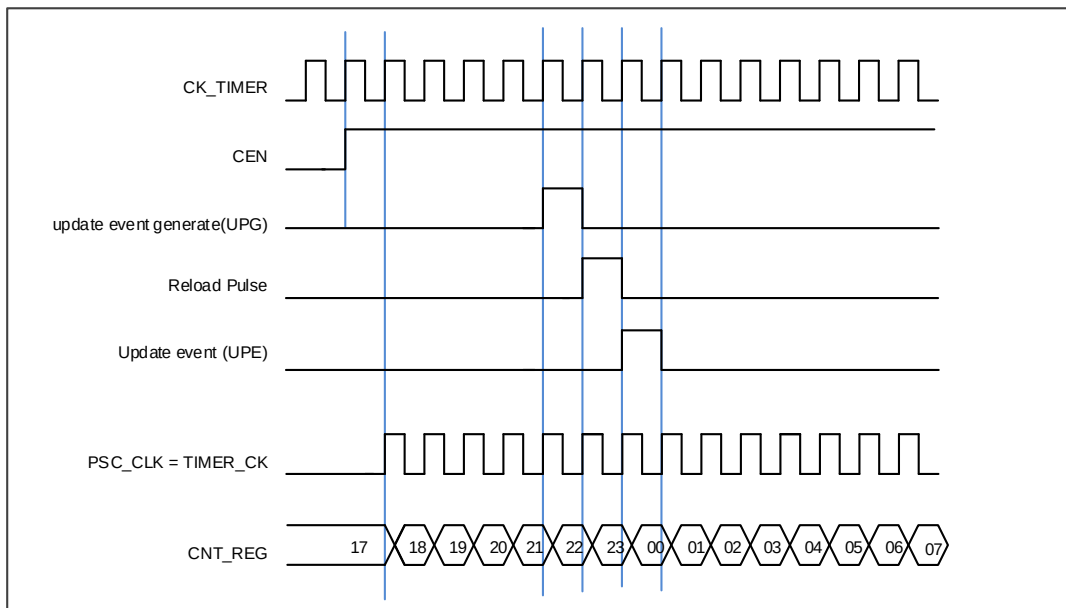
图 15-81. 内部时钟分频为 1 时正常模式下的控制电路
