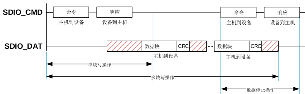
图 19-3. SDIO 多块写操作
