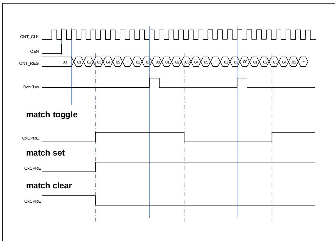
图 15-79. 三种输出比较模式
