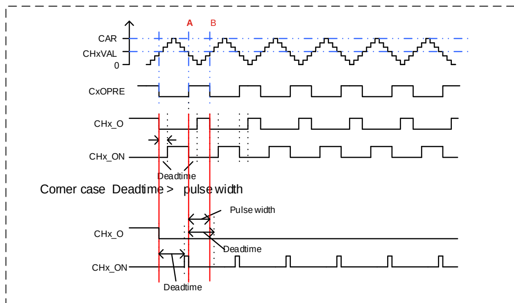
图 15-18. 带死区时间的互补输出
