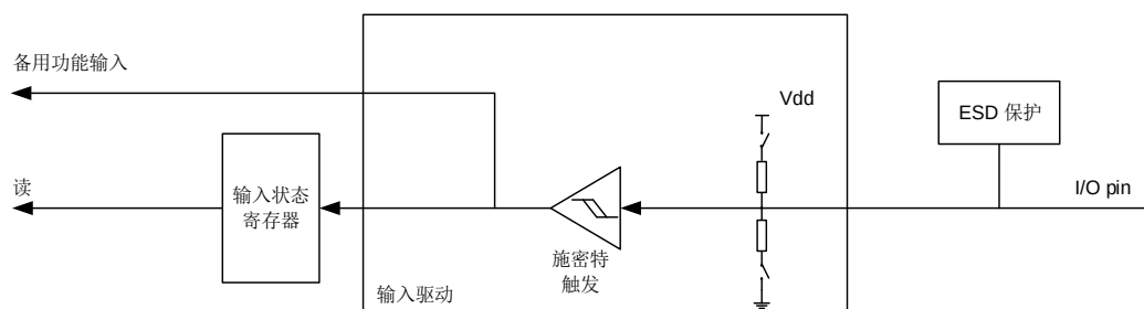
图 7-2. 输入配置
