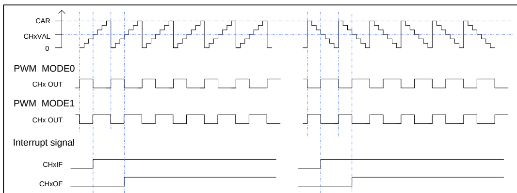
图 15-46. CAPWM 时序图
