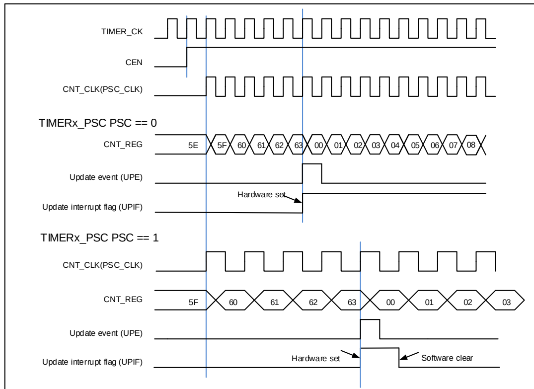
图 15-56. 向上计数时序图, PSC=0/1
