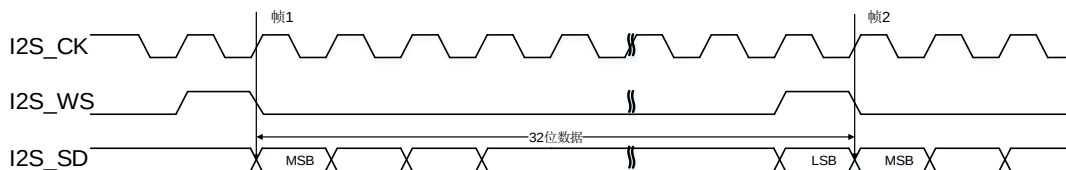
图 18-31. PCM 标准短帧同步模式时序图 (DTLEN=10, CHLEN=1, CKPL=1)
