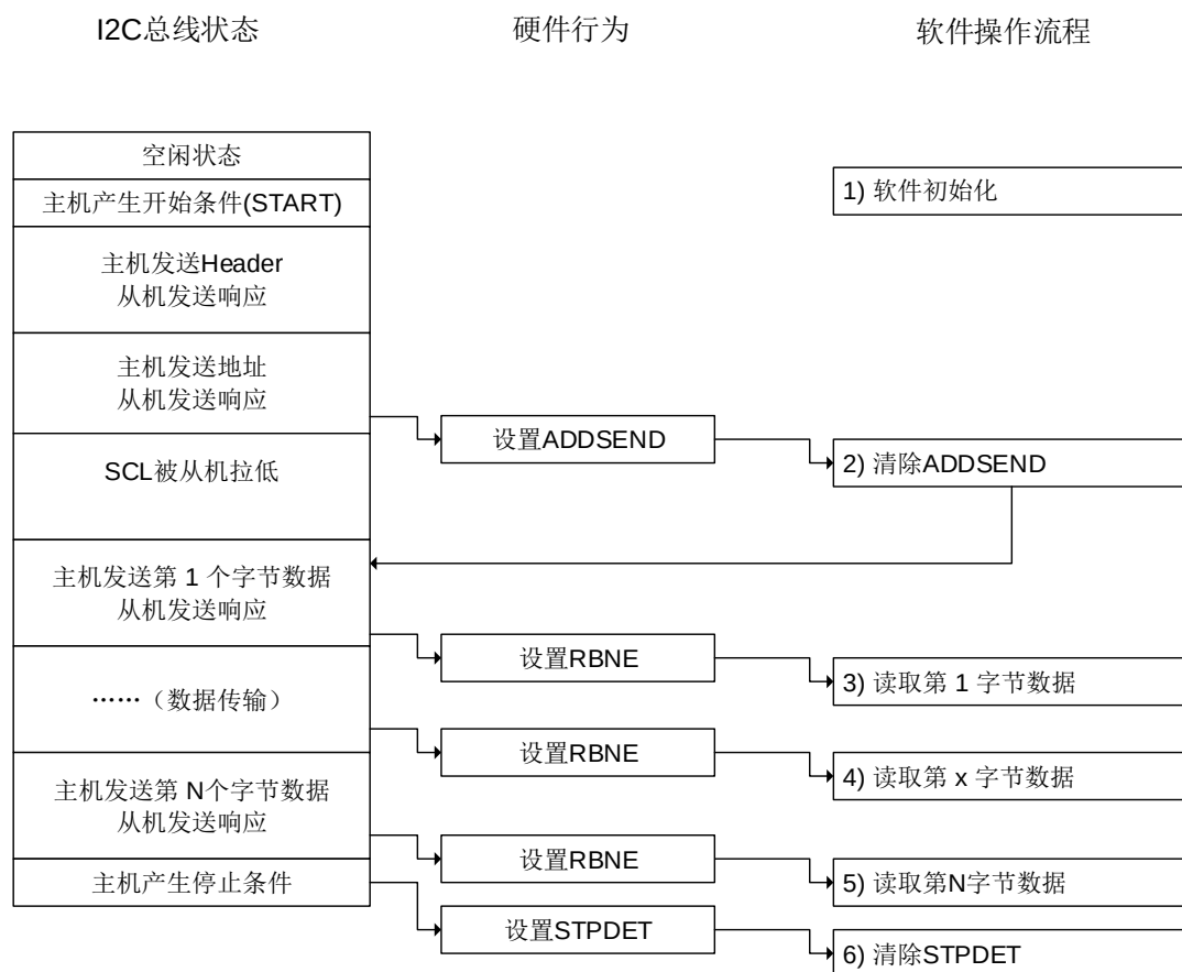
图 17-10. 从机接收模式（10 位地址模式）
