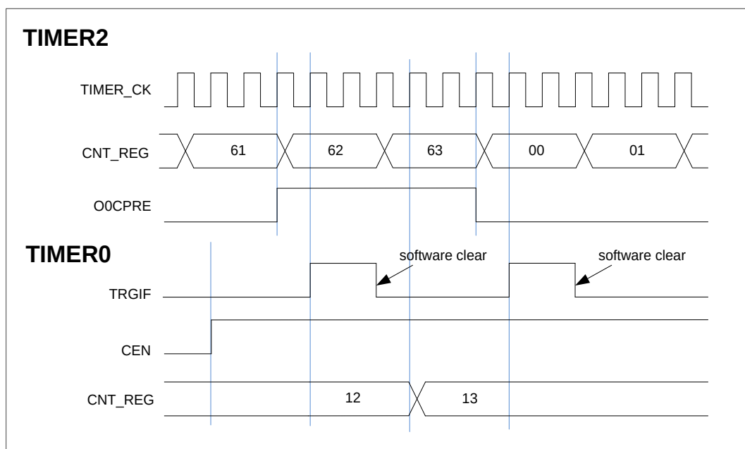
图 15-32. 用定时器 2 的 O0CPRE 信号选通定时器 1
