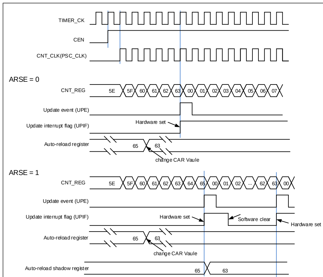
图 15-84. 向上计数时序图，在运行时改变 TIMERx_CAR 寄存器的值
