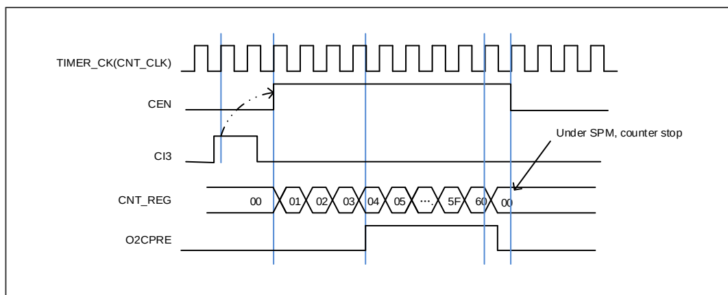
图 15-69. 单脉冲模式，TIMERx_CHxCV = 0x04 TIMERx_CAR=0x60
