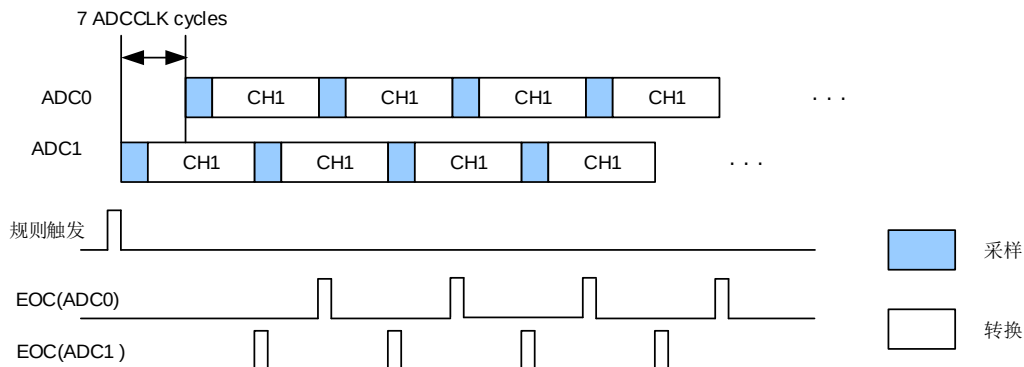
图 11-13. 一个采用连续转换模式通道上的快速交叉模式
