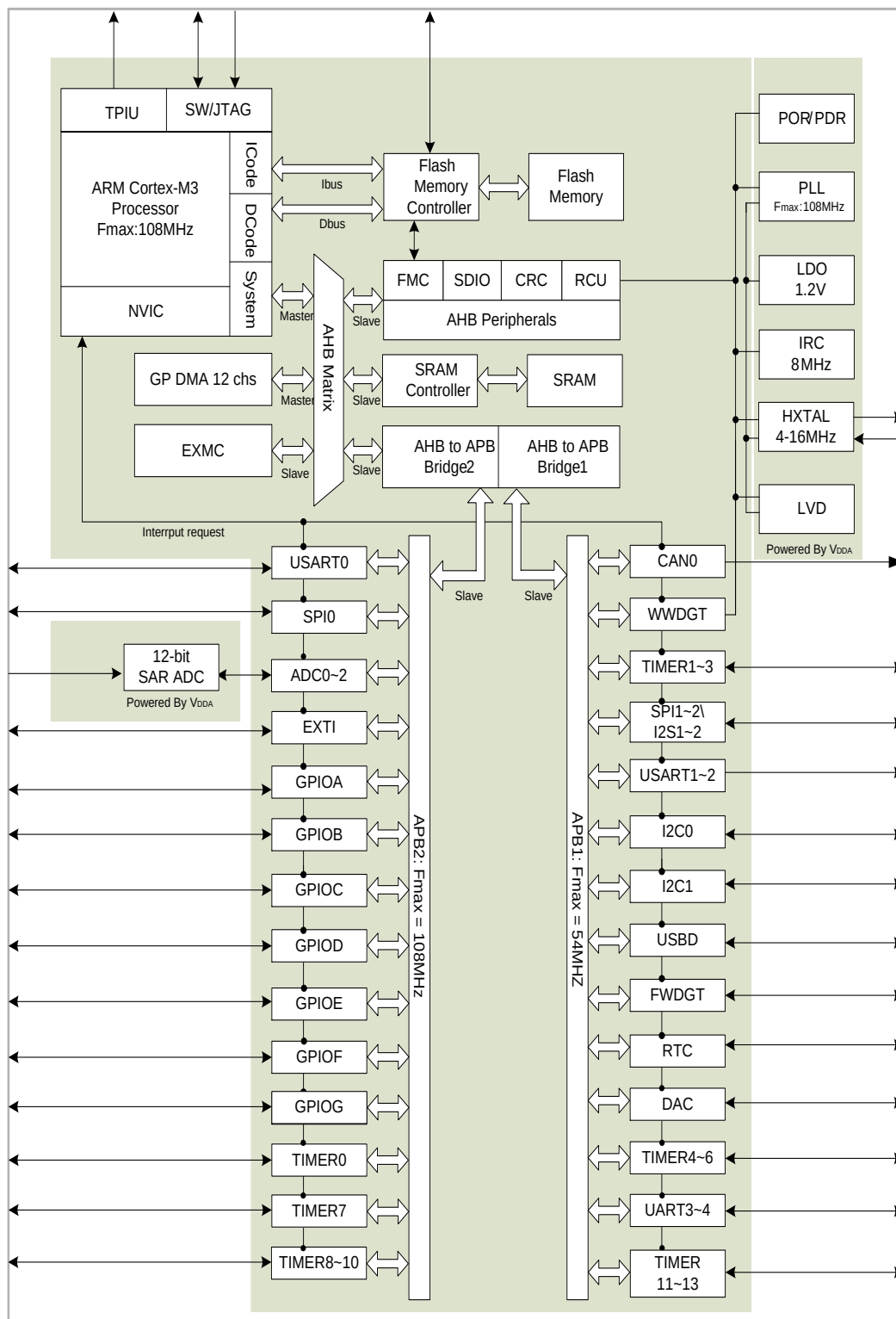
图 1-4. GD32F10x Extra-density 系列系统架构
