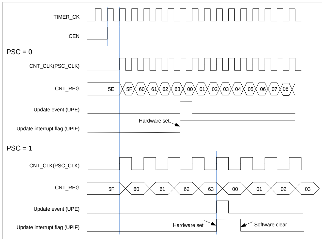
图 15-37. 向上计数时序图, PSC=0/1
