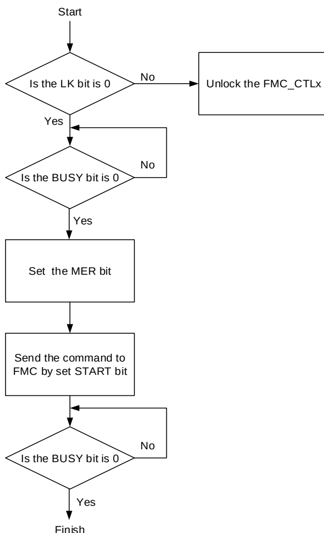
图 2-2. 整片擦除操作流程
