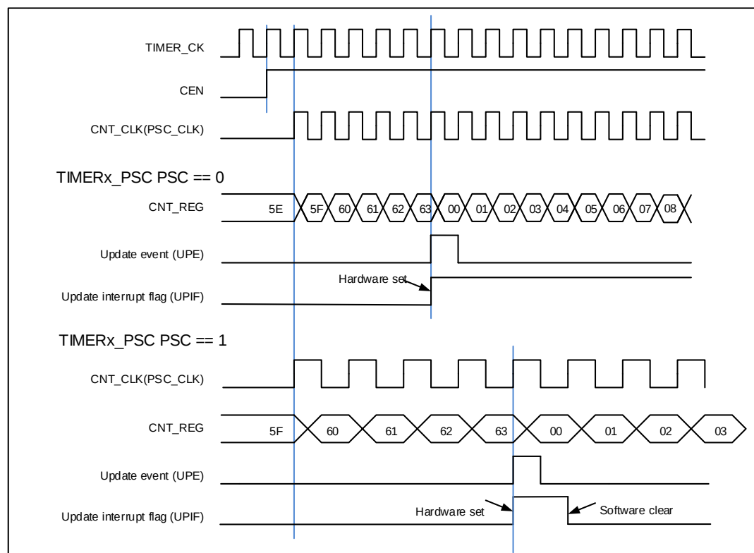
图 15-83. 向上计数时序图，PSC=0/1
