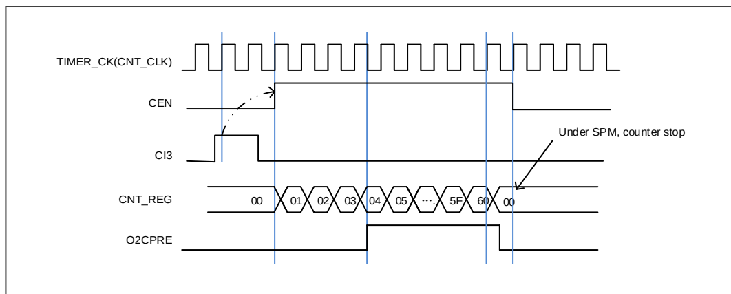
图 15-52. 单脉冲模式，TIMERx_CHxCV = 0x04 TIMERx_CAR=0x60
