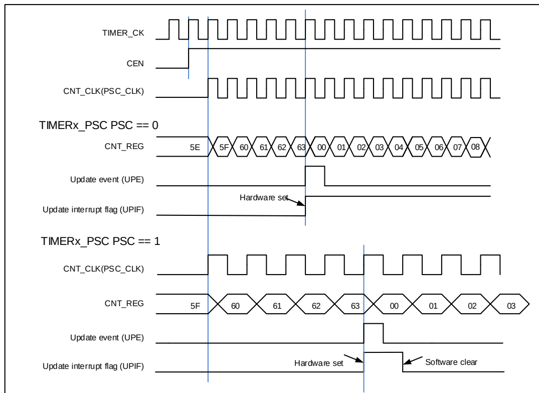
图 15-73. 向上计数时序图, PSC=0/1
