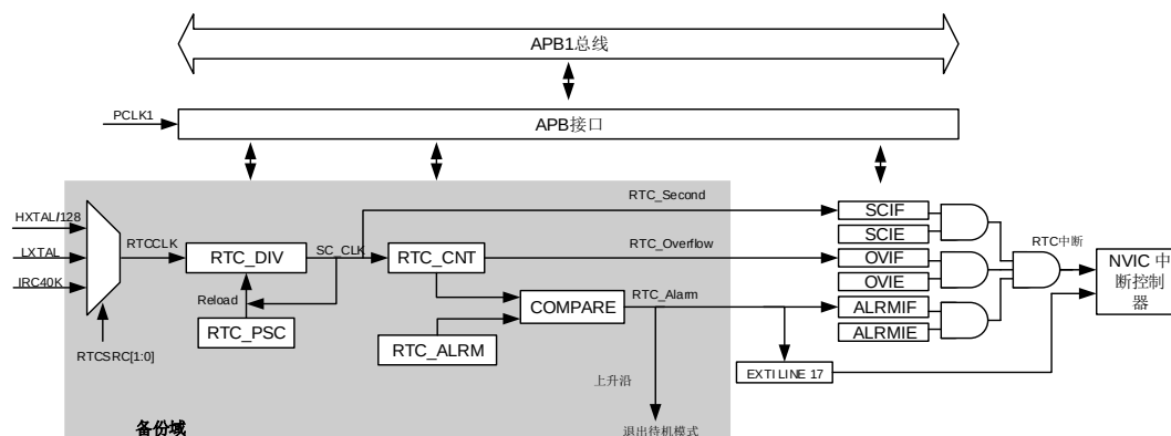
图 14-1. RTC 框图
