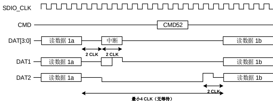
图 19-13. 使用 SDIO_DAT[2]信号线的读等待操作
