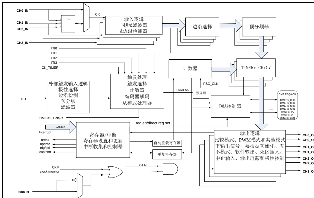
图 15-1. 高级定时器结构框图
