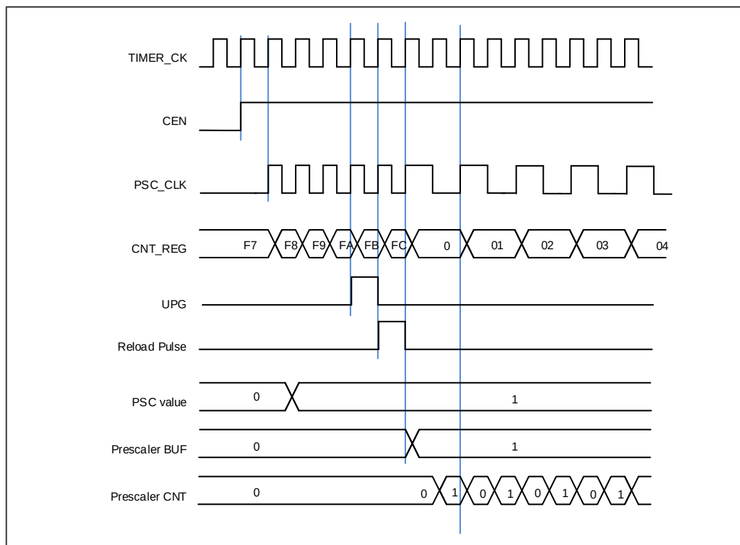
图 15-72. 当预分频器的参数从 1 变到 2 时，计数器的时序图
