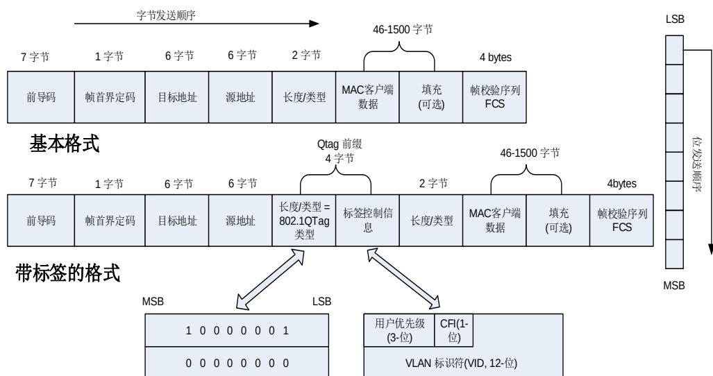
图 22-2. MAC/带标签的 MAC 帧格式
