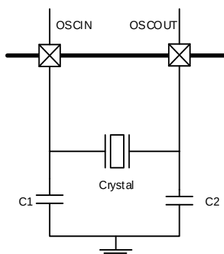
图5-3. HXTAL时钟源
