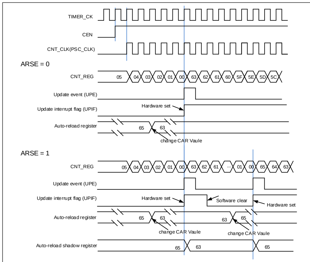
图 15-76. 向下计数时序图，在运行时改变 TIMERx_CAR 寄存器值
