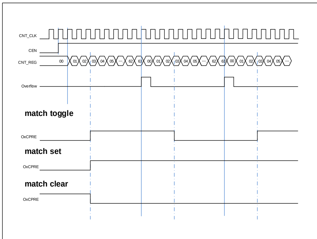
图 15-44. 三种输出比较模式
