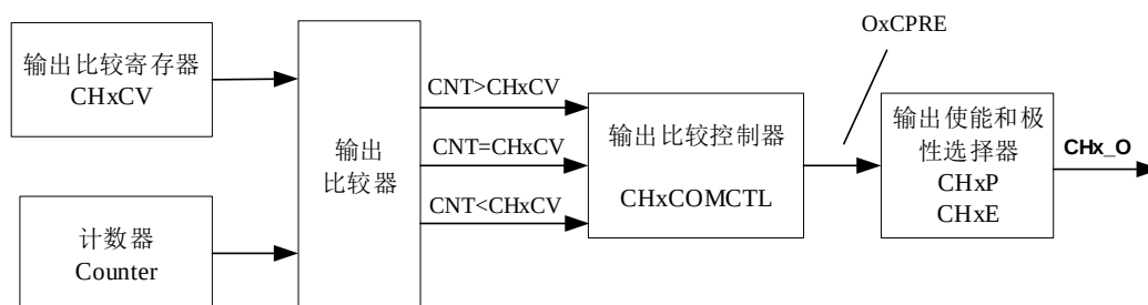
图 15-62. 输出比较逻辑 (x=0,1)
