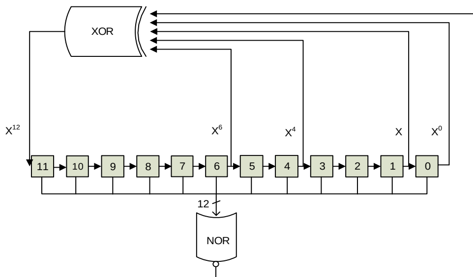
图 12-2. DAC LFSR 算法
