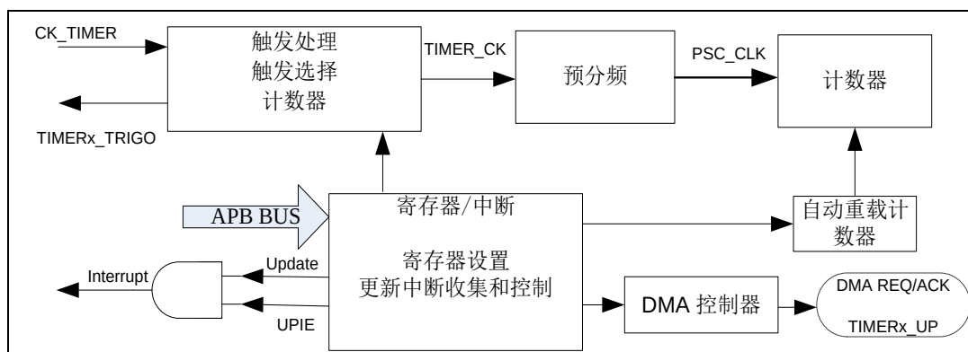
图 15-80. 基本定时器结构框图
