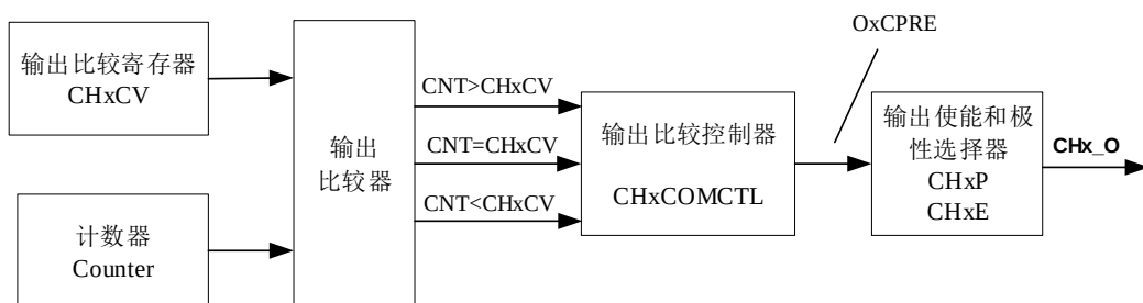
图 15-43. 输出比较逻辑 (x=0,1,2,3)
