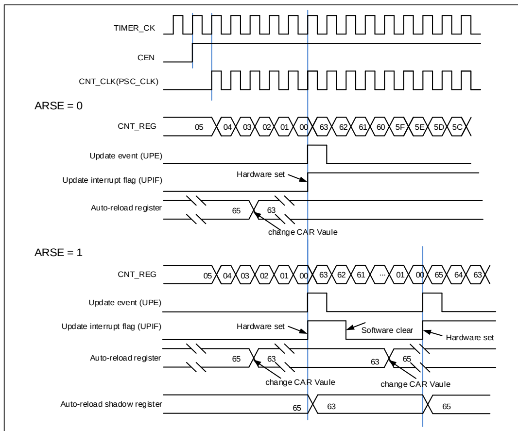
图 15-59. 向下计数时序图，在运行时改变 TIMERx_CAR 寄存器值
