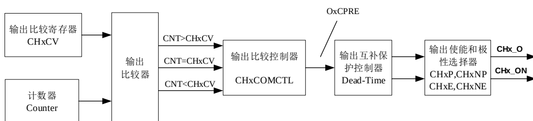
图 15-14. 输出比较逻辑
