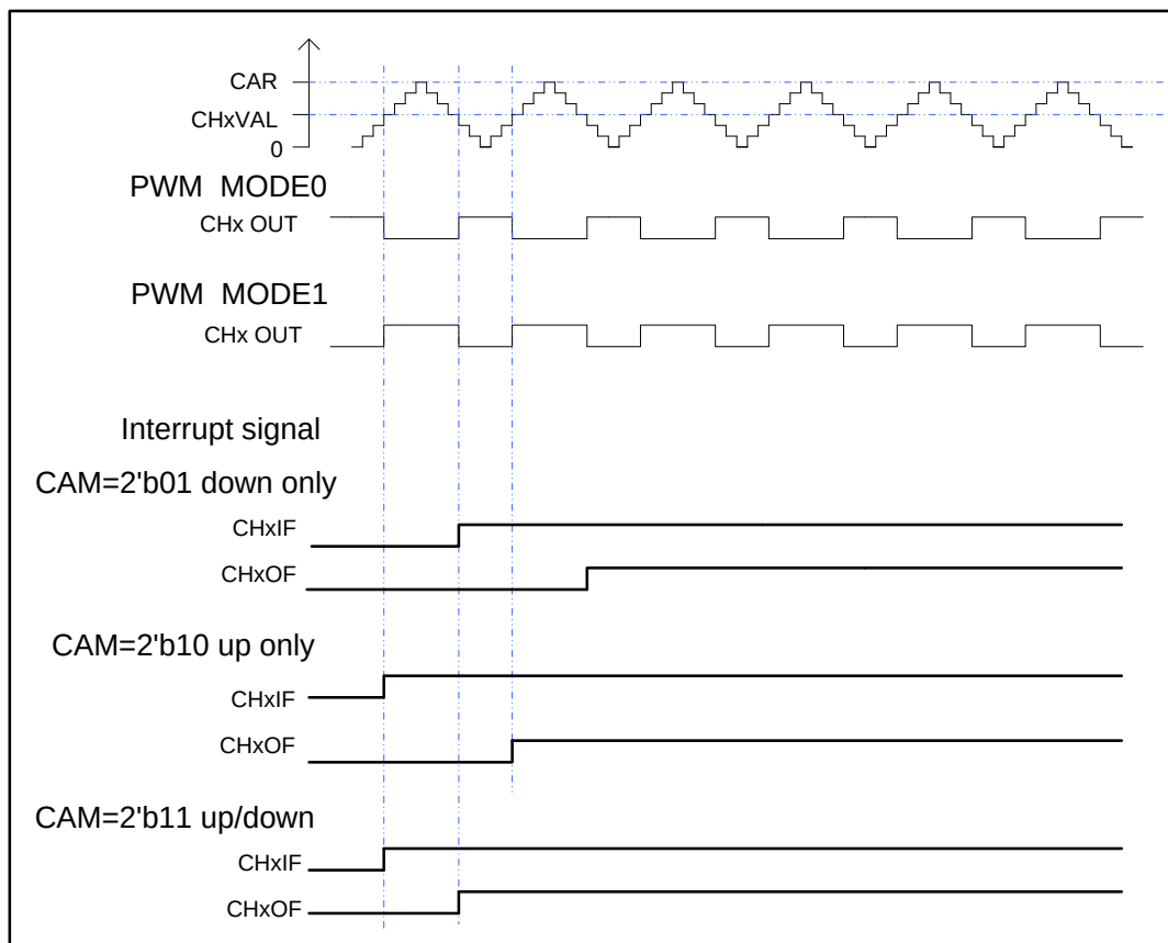
图 15-65. CAPWM 时序图
