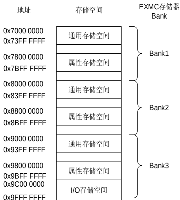
图 20-4. NAND/PC Card 地址映射
