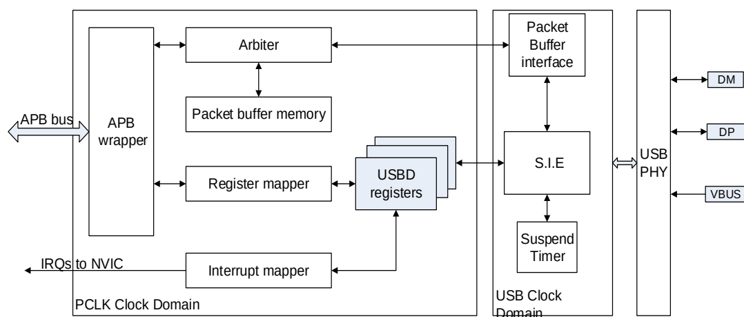
图 23-1. USB D 模块图
