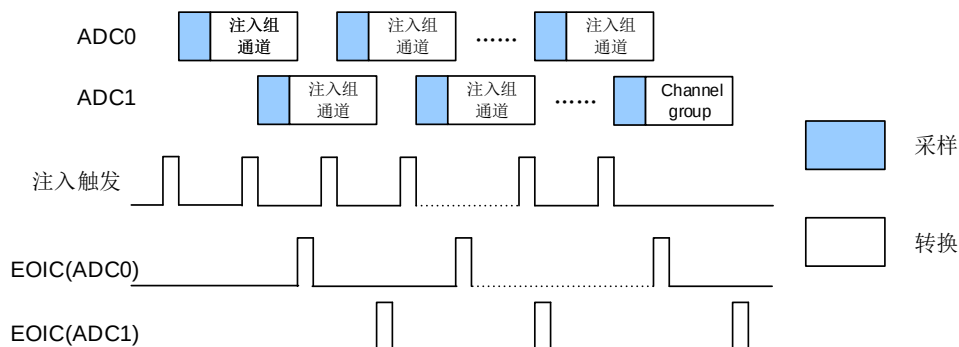
图 11-15. 交替触发: 注入通道组
