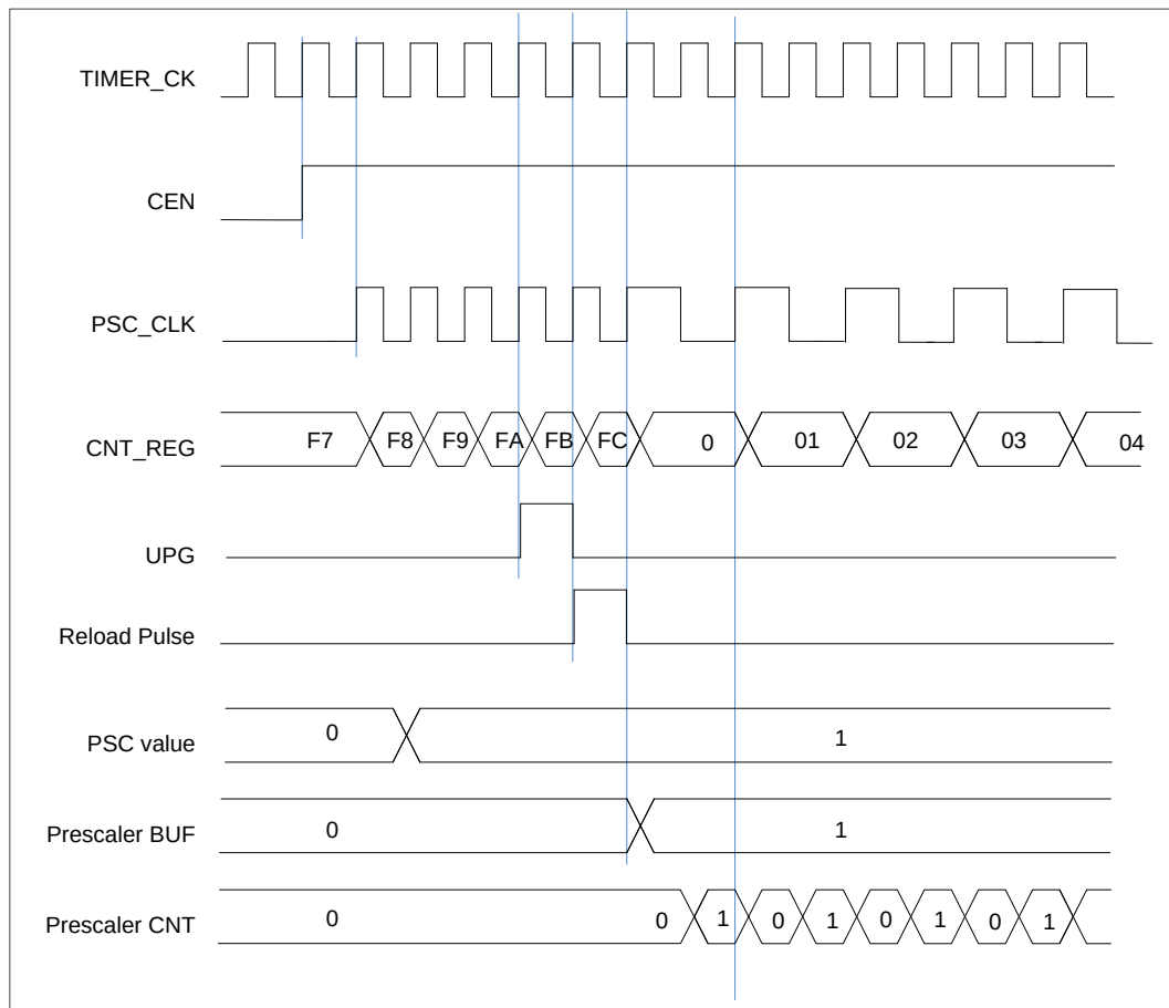
图 15-3. 当预分频器的参数从 1 变到 2 时，计数器的时序图
