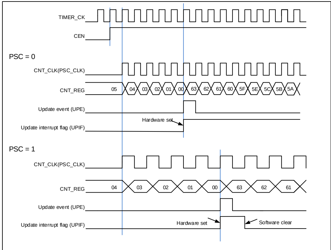
图 15-75. 向下计数时序图, PSC=0/1
