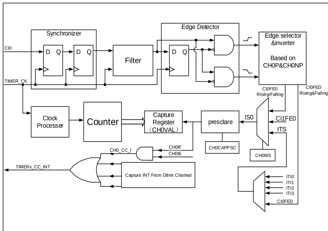
图 15-42. 输入捕获逻辑
