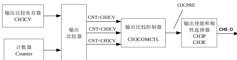
图 15-14. 输出比较逻辑
