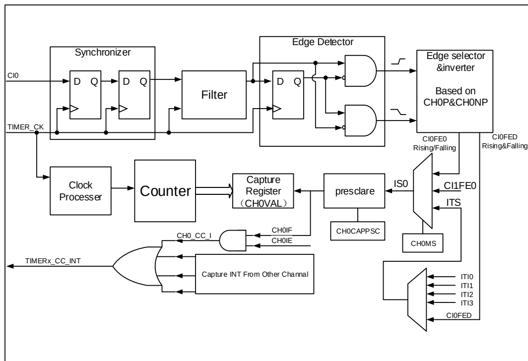
图 15-78. 输入捕获逻辑
