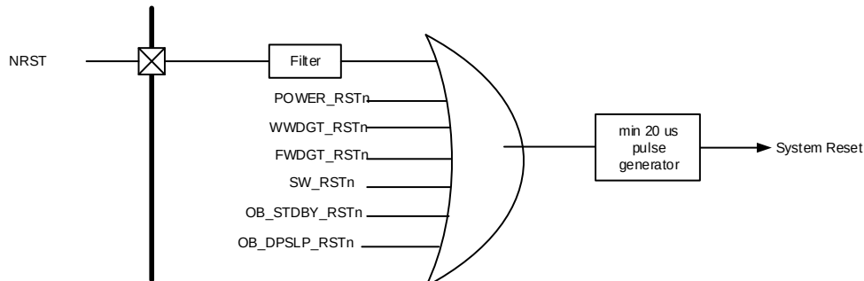
图5-5. 系统复位电路
