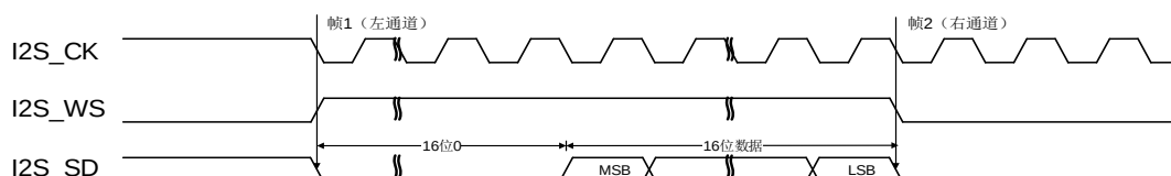
图 18-27. LSB 对齐标准时序图 (DTLEN=00, CHLEN=1, CKPL=1)
