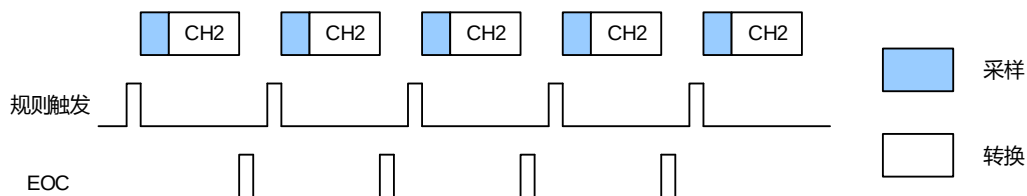
图 11-2. 单次转换模式
