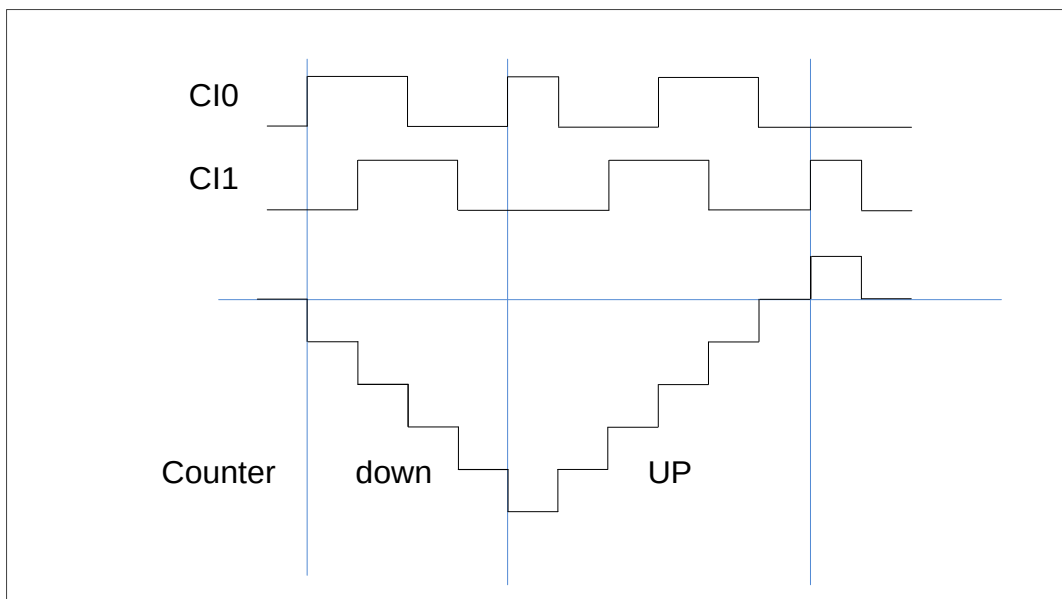
图 15-21. CI0FE0 极性反相的编码器接口模式下的例子
