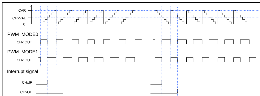
图 15-16. EAPWM 时序图
