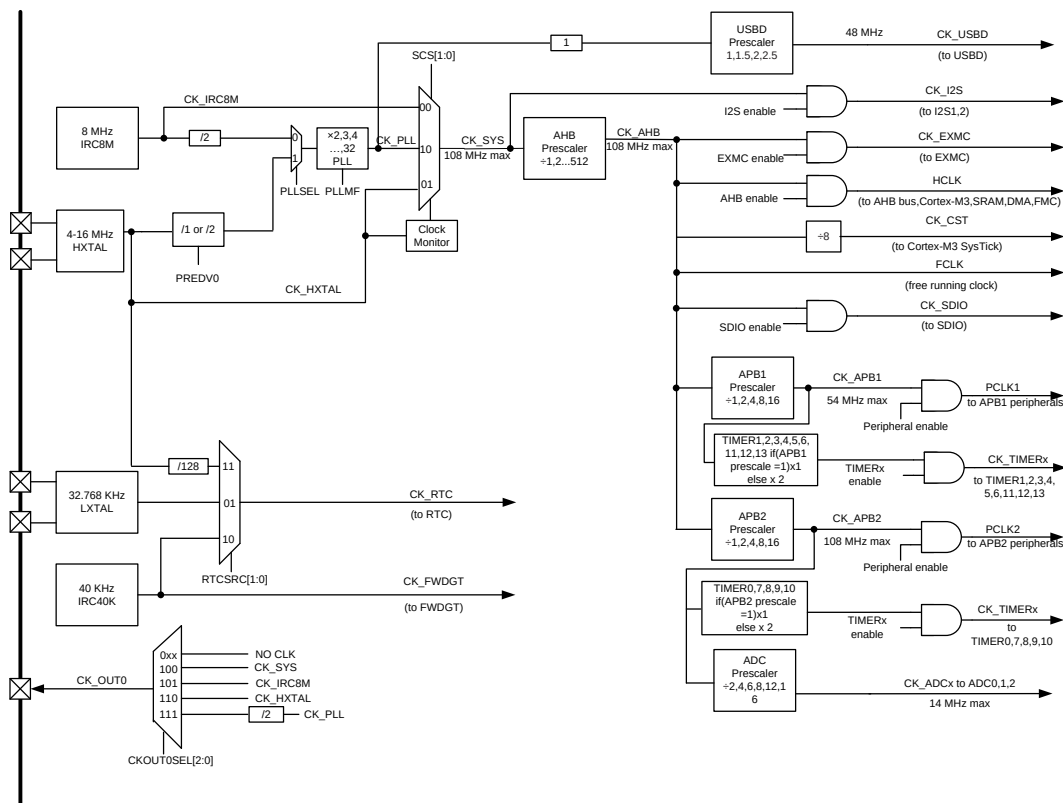
图5-2. 时钟树
