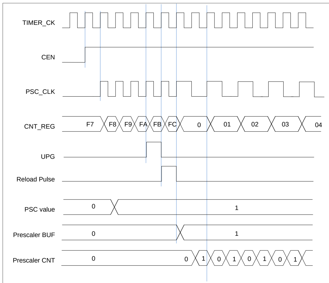
图 15-55. 当预分频器的参数从 1 变到 2 时，计数器的时序图
