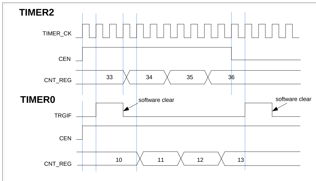
图 15-31. 用定时器 2 的使能来选通定时器 0
