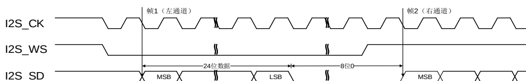
图 18-13. I2S 飞利浦标准时序图 (DTLEN=01, CHLEN=1, CKPL=1)
