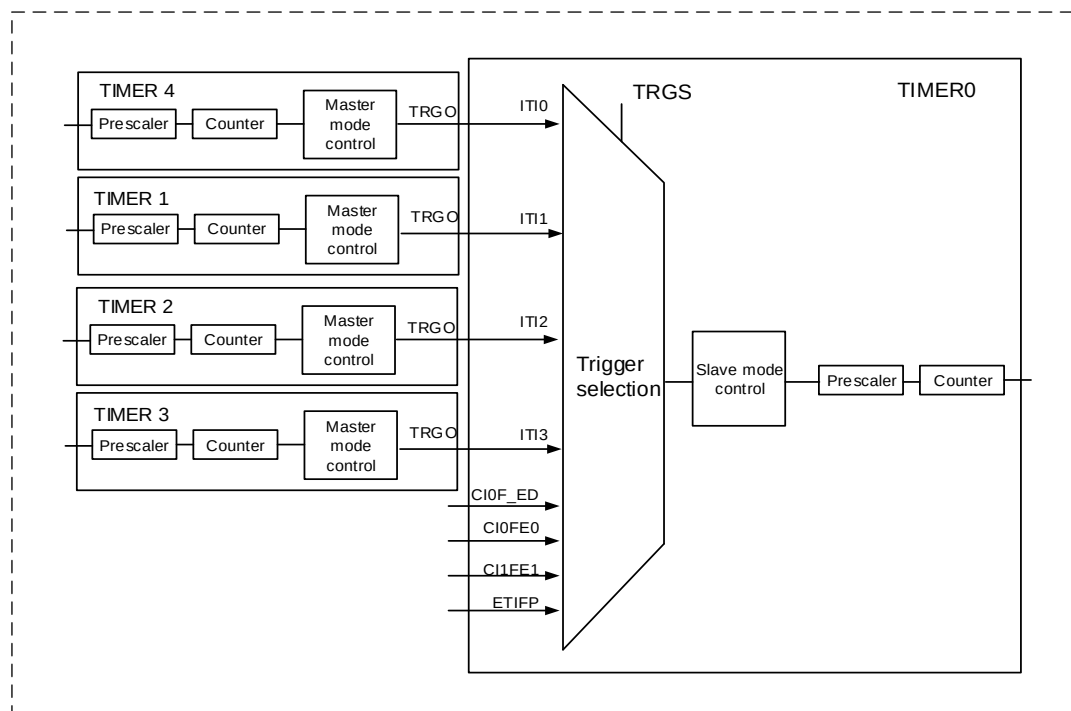
图 15-28. 定时器 0 主/从模式的例子
