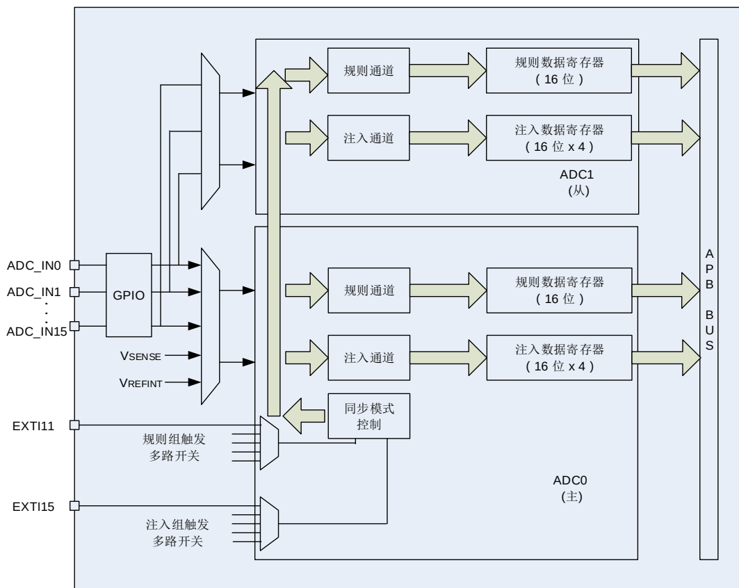
图 11-10. ADC 同步框图
