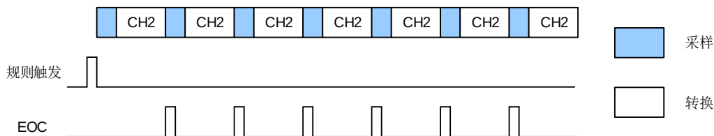
图 11-3. 连续转换模式
