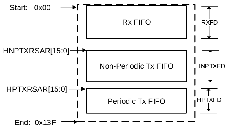
图 24-5. 主机模式 FIFO 空间
