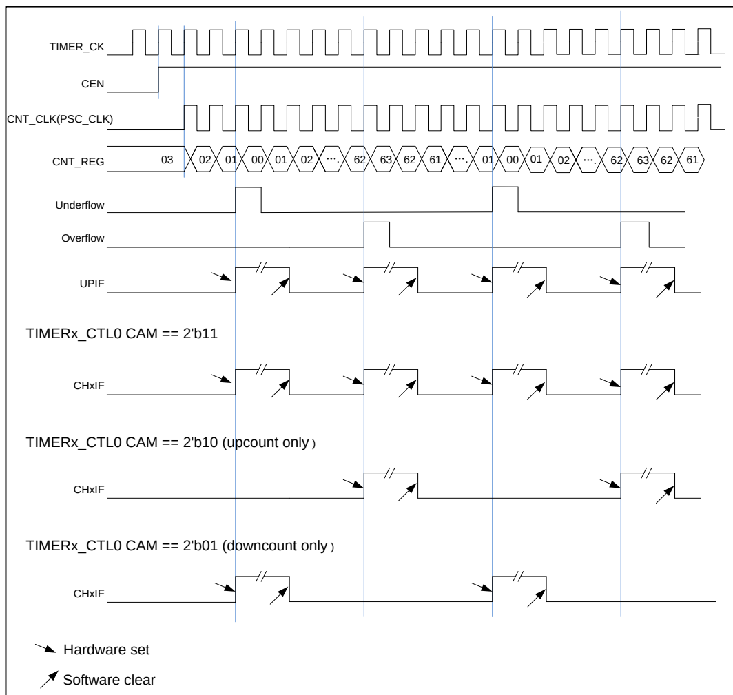
图 15-41. 中央对齐计数模式计数器时序图
