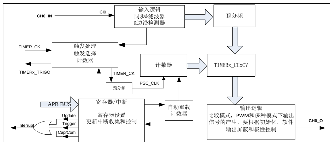
图 15-70. 通用定时器 L2 结构框图
