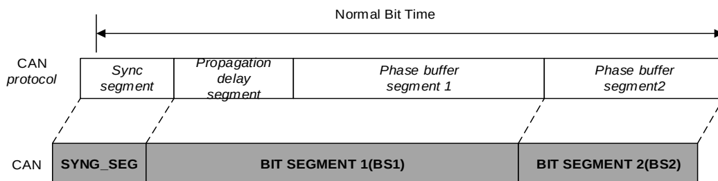
图 21-11. 位时序
