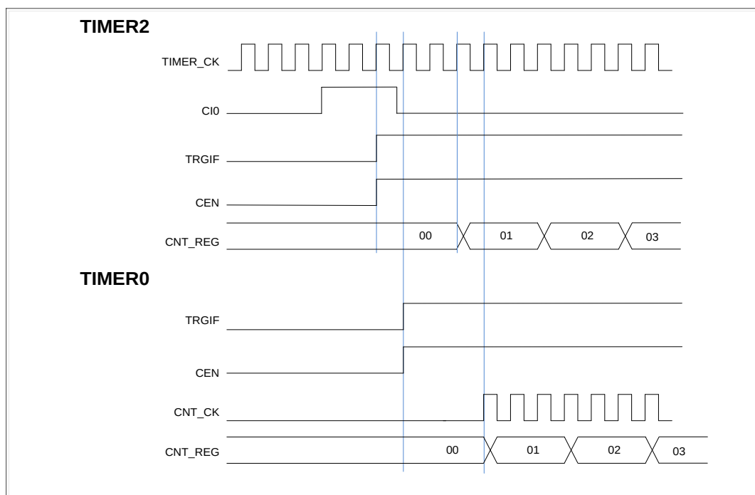
图 15-33. 用定时器 2 的 CI0 输入来触发定时器 0 和定时器 2
