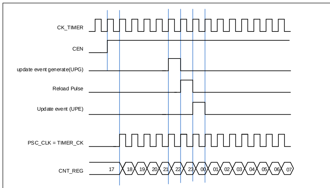
图 15-71. 内部时钟分频为 1 时正常模式下的控制电路
